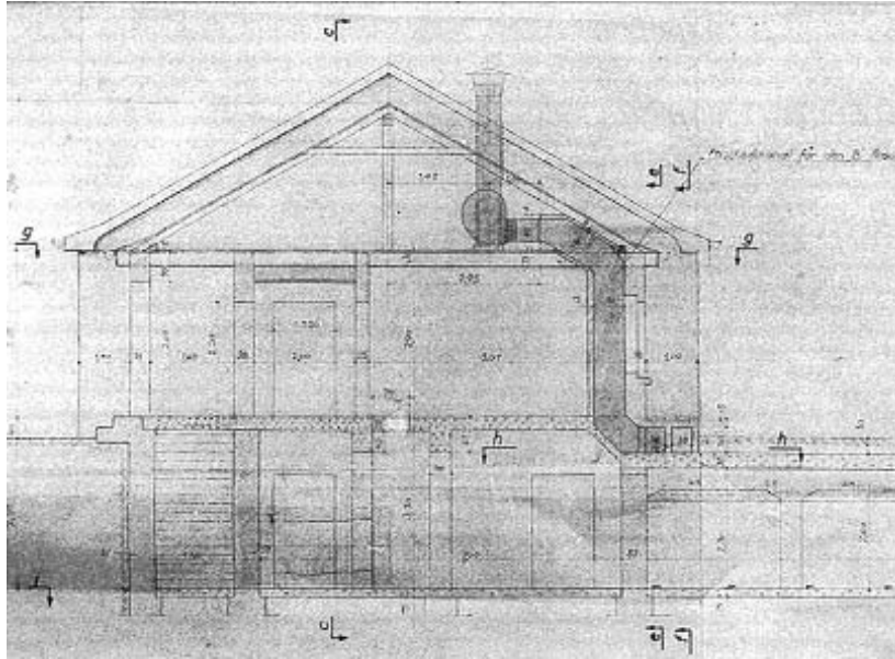
Coupe de la chambre à gaz du crématoire II, établie en 1941 par l'entreprise Topf.
